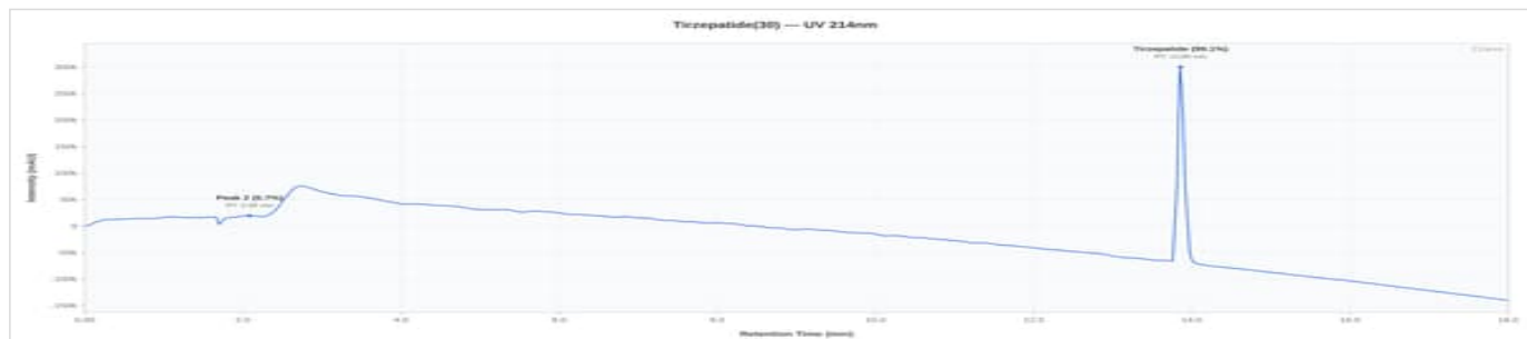
Tirzepatide 30 - ZRV-TRZ30-001: UV Chromatogram
